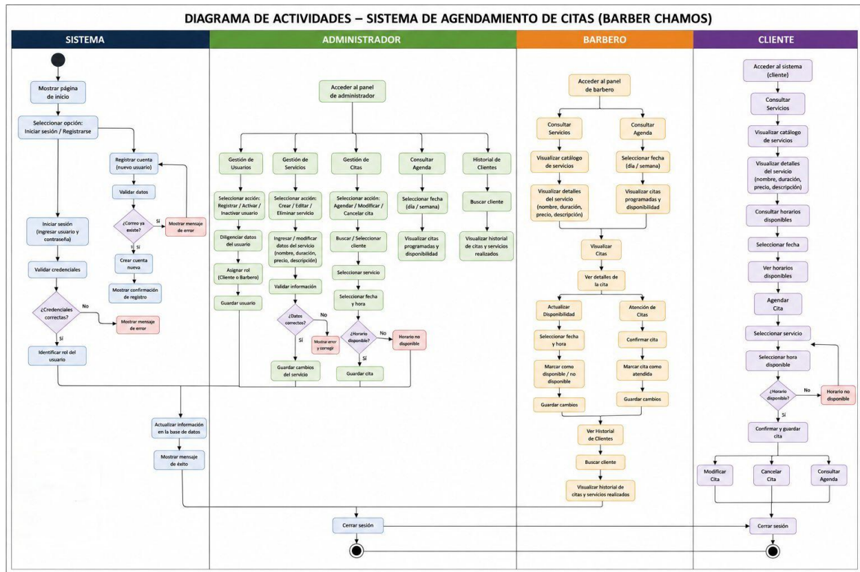
diagrama 1 diagrama de actividades
