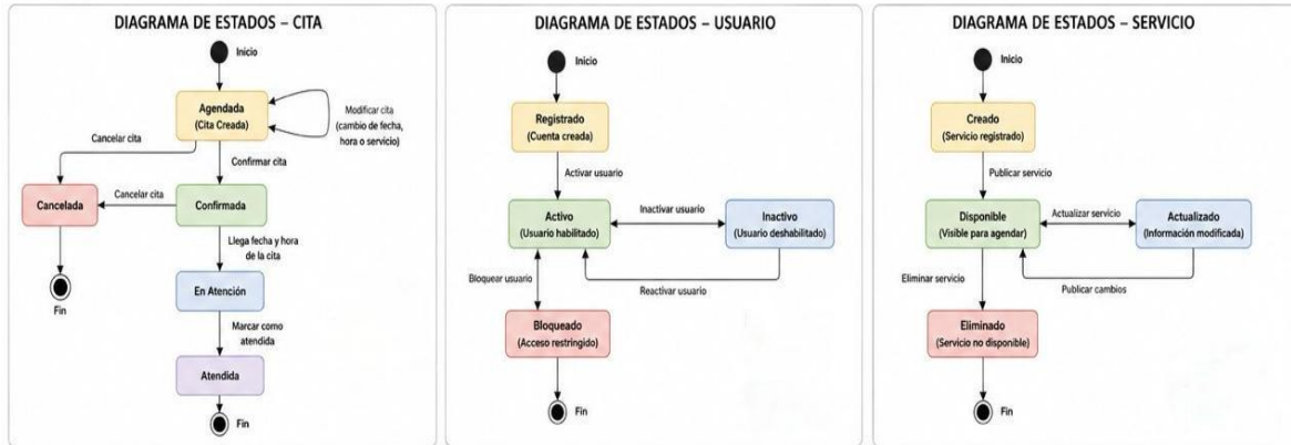
diagrama 2 diagrama de estado
