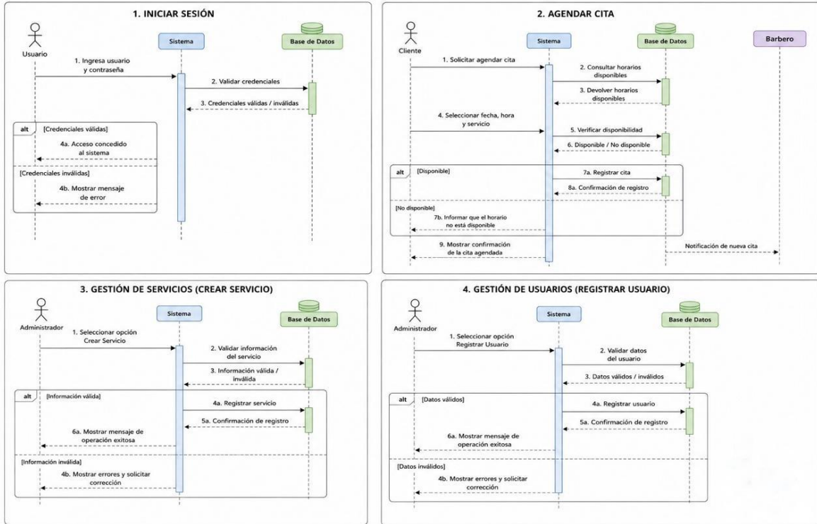
diagrama 3 diagramas de secuencia
